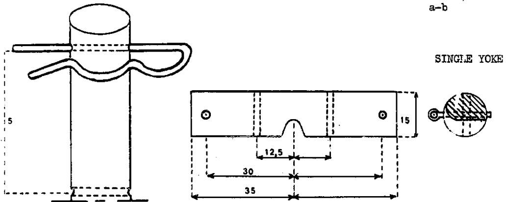
Fig. 38 - LONG YOKE
