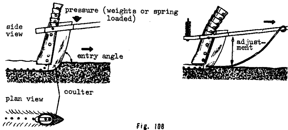
Hoe coulter
