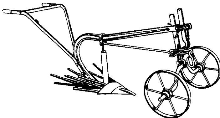
Fig. 154 · Potato lifter
